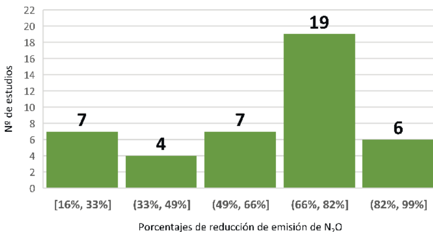
FIGURA 2 Histograma de la efectividad de los inhibidores de la nitrificación DMPP y DMPSA en reducir las emisiones de óxido nitroso ( N_2O ).
